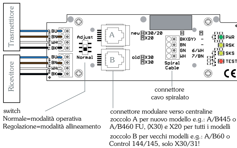
2x M16 1x M20 per connettore modulare
